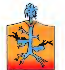
розігріті гірські породи Гейзер Бурхливий витік гарячої води і пари, спричинений вулканічним теплом
